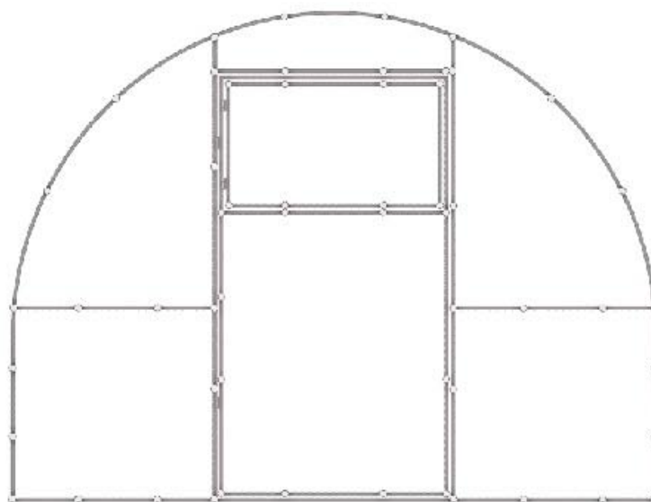
JOON. 2. POLÜKARBONAADI KINNITAMINE KASVUHOONE OTSASEINAL
